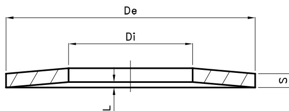
ARANDELA CONICA ELASTICA
