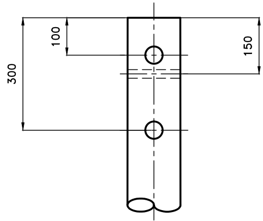
Detalle de Agujeros Pasantes
