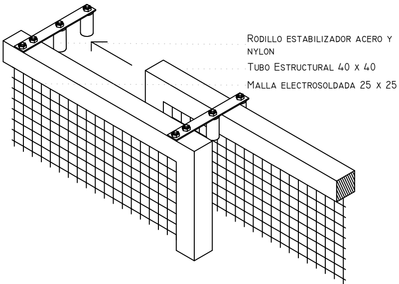
DETALLE RODILLOS SUPERIORES PUERTAS CORREDIZAS
