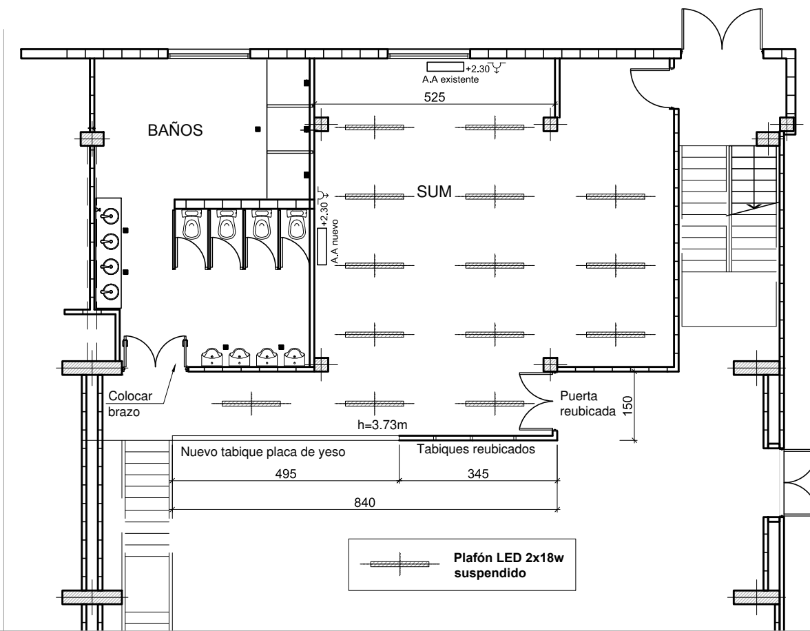
Planta sector Montaje SET - PROYECTO Esc 1:100
