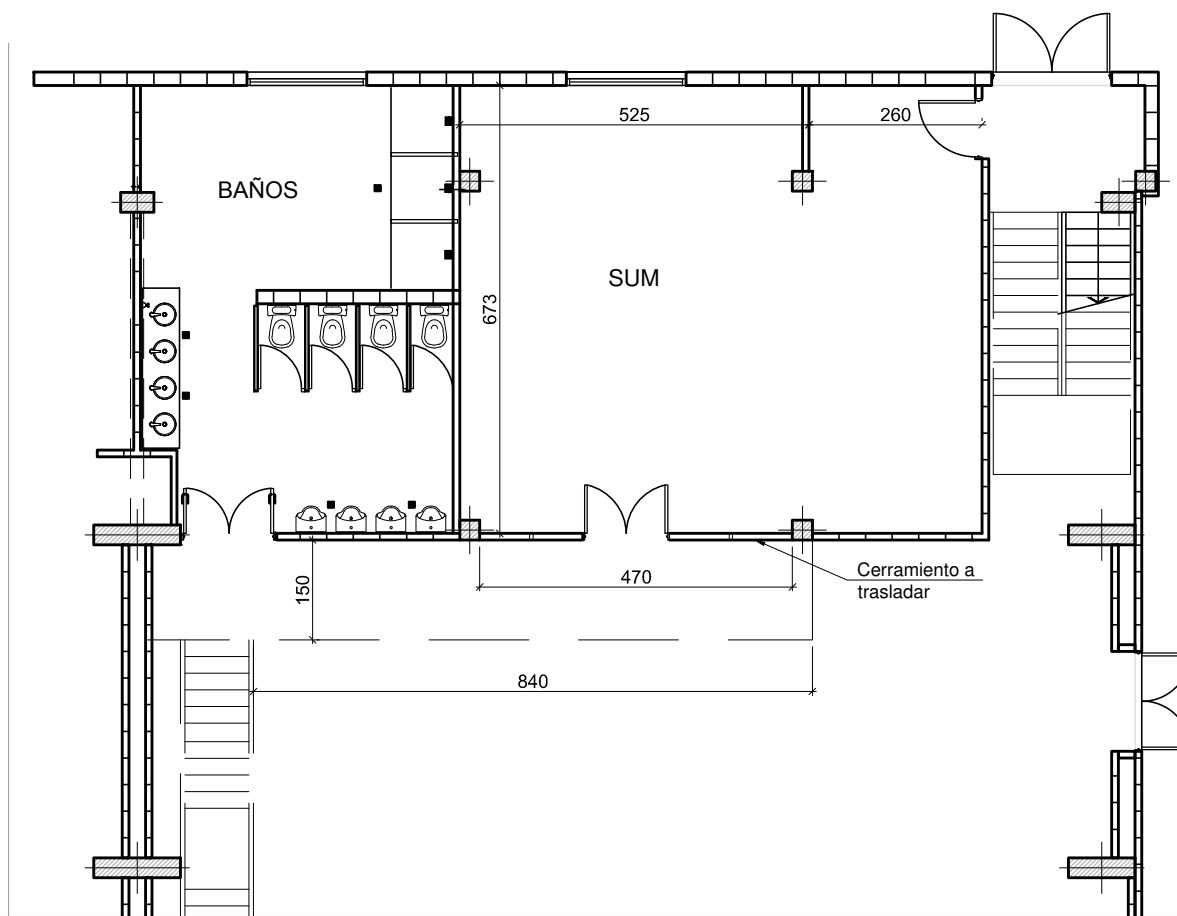
Planta sector Montaje SET - EXISTENTE Esc 1:100
