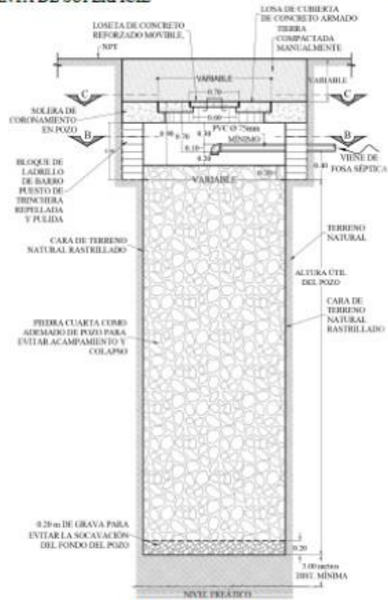
VISTA EN ELEVACIÓN
